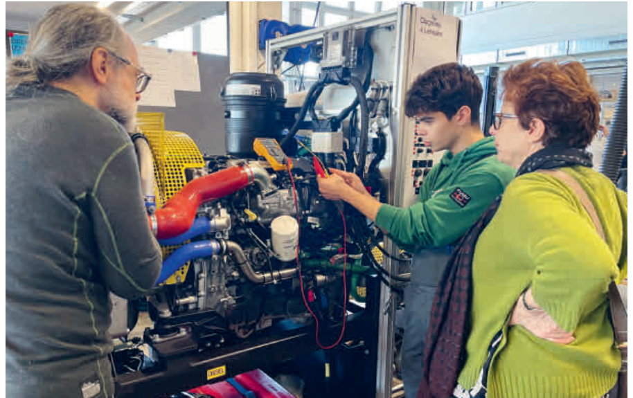
Ein Mechatronik-Lernender zeigt den Gästen am asb-Herbstanlass an einem Duro-Motor, wie man einen Spannungsfehler diagnostiziert und behebt.
